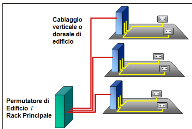
Figura 2 - Cablaggio verticale
